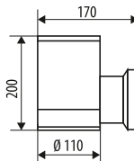
RINO S 608 Ø 110
